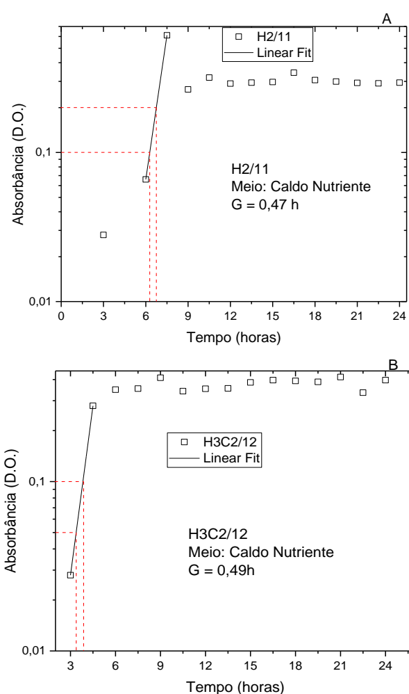
Figura 17: Cálculo do tempo de geração para as amostras de E. coli , em meio de caldo nutriente, através do gráfico de Absorbância em escala logarítmica. (A) H2/11: 0,47 horas; (B) H3C2/12: 0,49horas.
