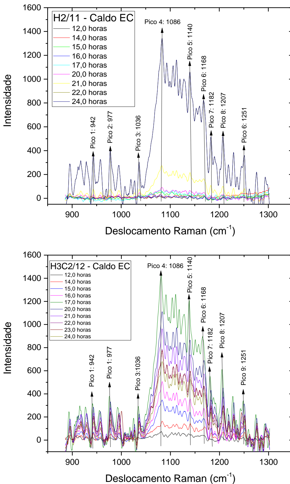
Figura 22: Espectros Raman sobrepostos ao longo de 24 horas para cepas de E. coli : amostras H2/11 e H3C2/12 em caldo EC. As setas indicam picos identificáveis
