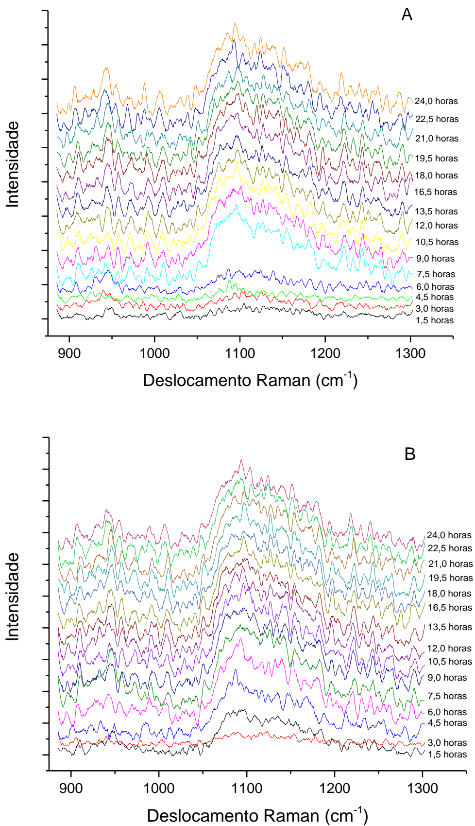
Figura 20: Espectros Raman ao longo de 24 horas para cepas de E. coli crescidas em caldo nutriente. A) Amostra H2/11. B) Amostra H3C2/12. Os espectros estão deslocados em 'y' para facilitar a visualização.
