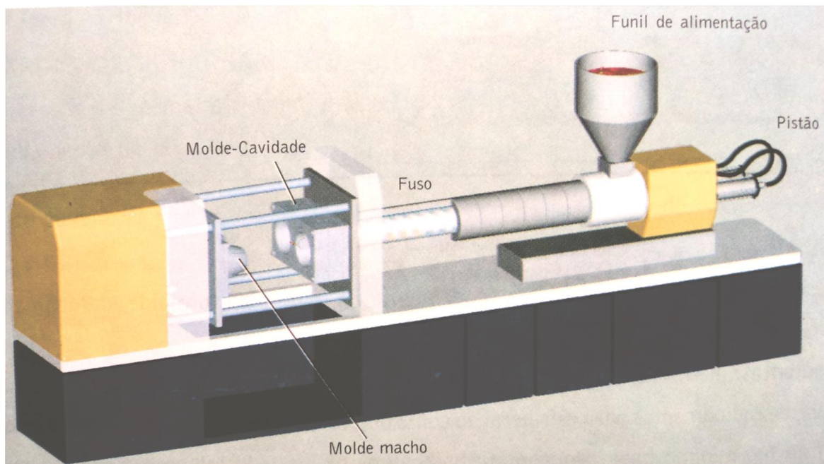
Figura 62: Processo de injeção. Fonte: Lima, 2006.
