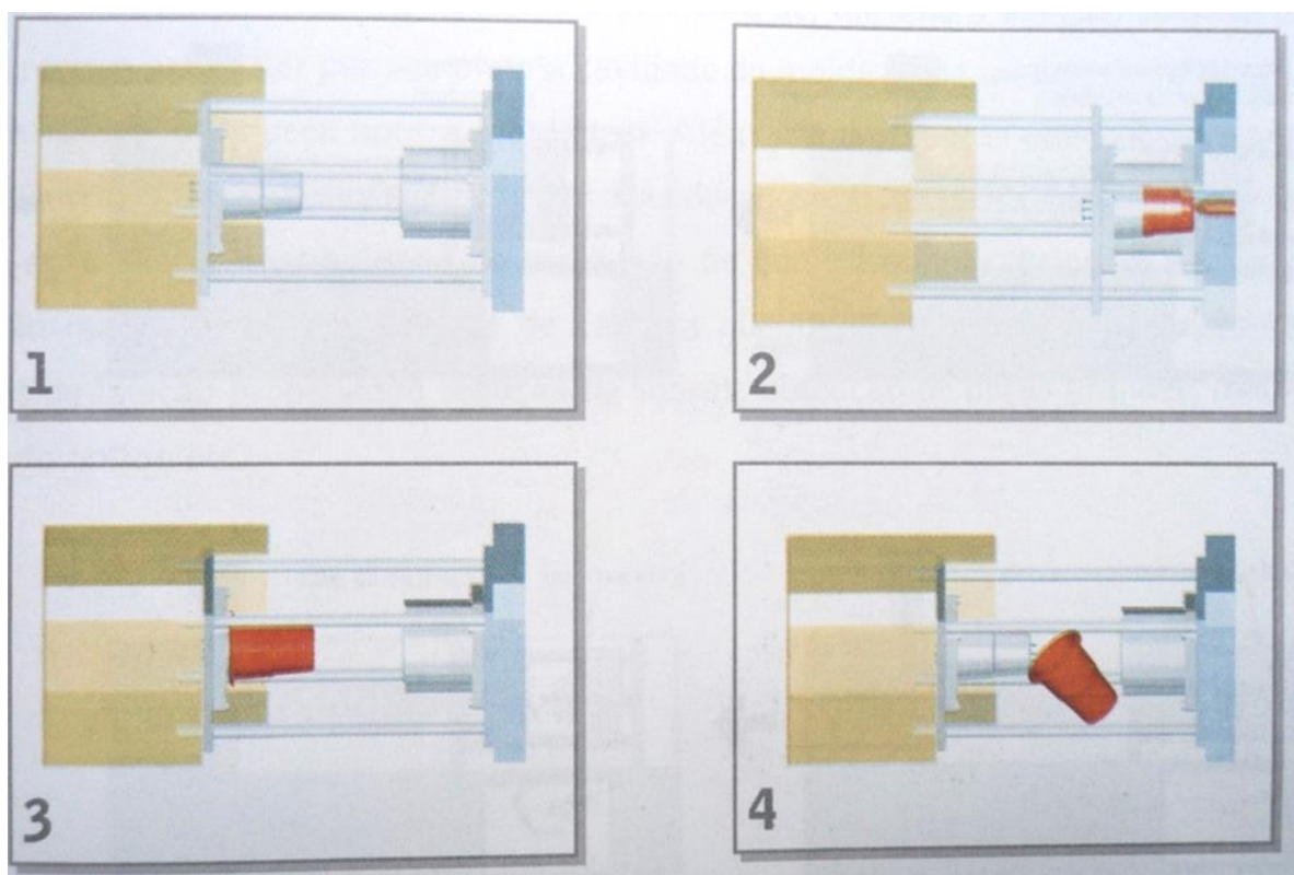
Figura 63: Processo de injeção Fonte: Lima, 2006.
