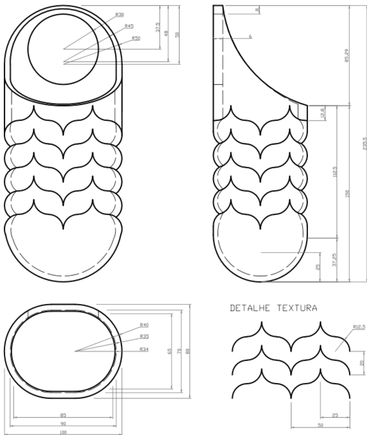
Figura 59: Desenho técnico do produto. Fonte: Autoria Própria
