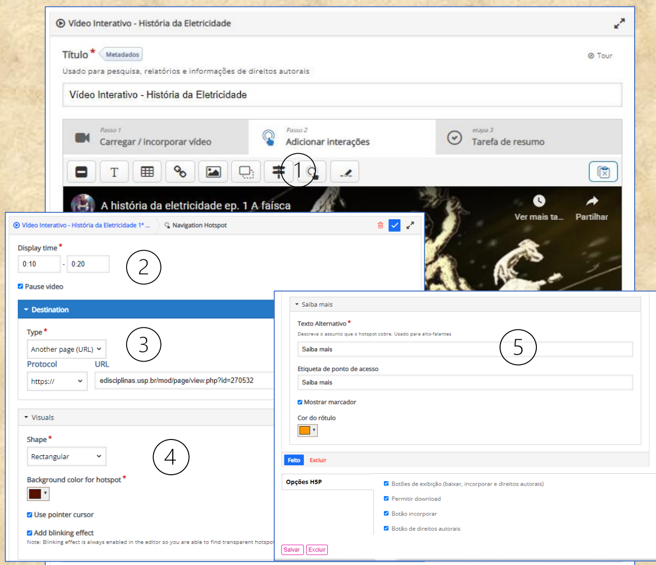
Figura 23 – Tela de configurações – Autoria própria
