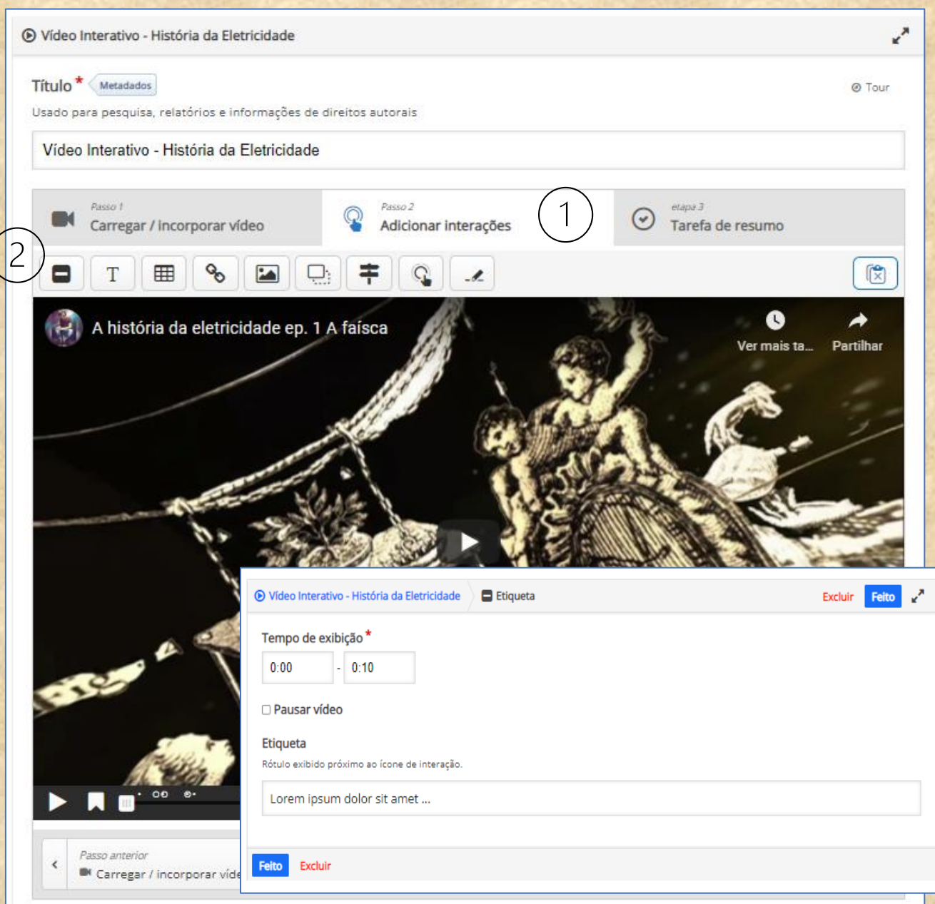
Figura 15 – Tela de configurações – Autoria própria
