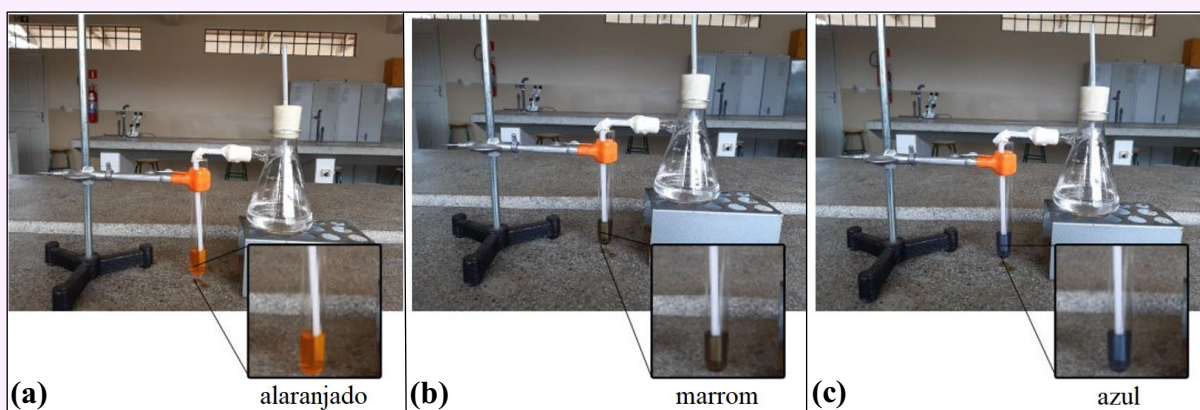
Figura 13: Etapas de coloração na reação do dicromato de potássio em meio fortemente ácido com etanol: (a) coloração alaranjada, apenas dicromato em meio fortemente ácido; (b) coloração marrom, início da reação com etanol e (c) verde-azulada, em que o cromo foi reduzido a cromo (II) ( Fonte: autoria própria)
