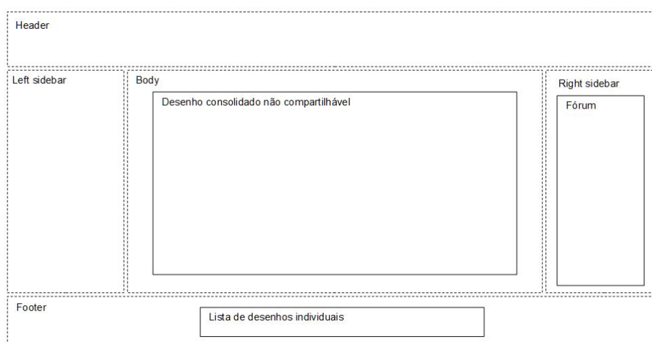
Figura 24 – Oficina C: wireframe referente à IU da fase de brainstorming gerado a partir dos desenhos consolidados.
