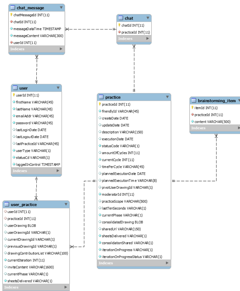
Figura 43 – Modelo do banco de dados do Sistema Design Participativo em Ação.
