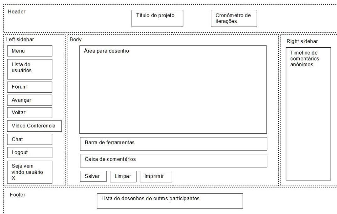
Figura 25 – Oficina C: wireframe referente à IU da fase de execução gerado com os resultados dos desenhos consolidados de todos os grupos da Oficina C.
