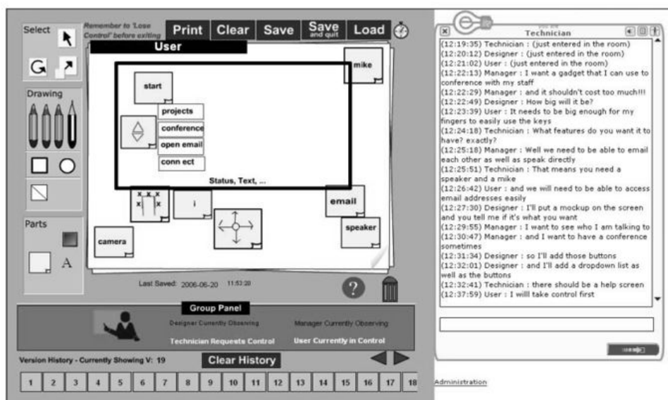
Figura 10 – Interface de usuário (IU) da ferramenta PICTIOL.
