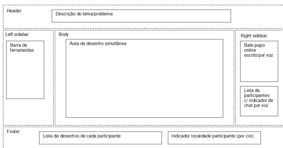
Figura 28 – Oficina A, B e C: wireframe referente à IU da fase de consolidação.
