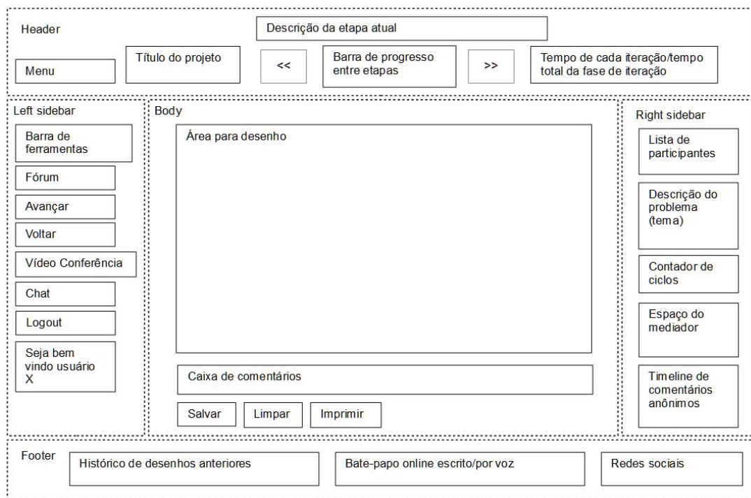
Figura 27 – Oficina A, B e C: wireframe referente à IU da fase de execução.
