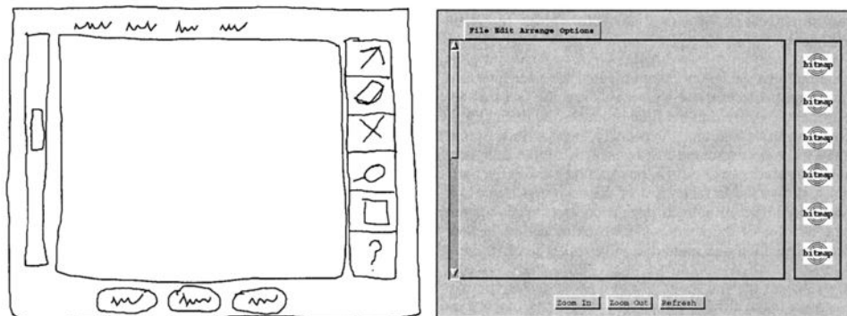
Figura 5 – Do lado esquerdo, o sketch produzido utilizando o pad eletrônico e stylus . Do lado direito, a interface resultante após a transformação.
