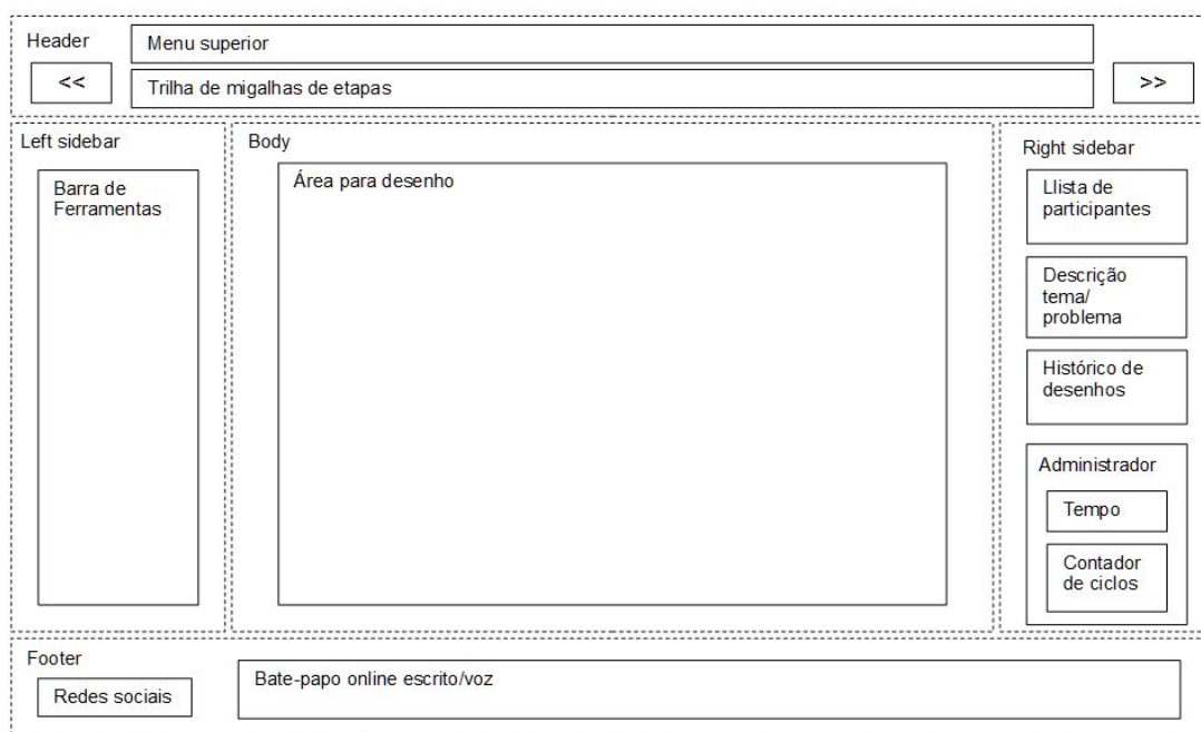
Figura 19 – Oficina B: wireframe referente à IU da fase de execução.
