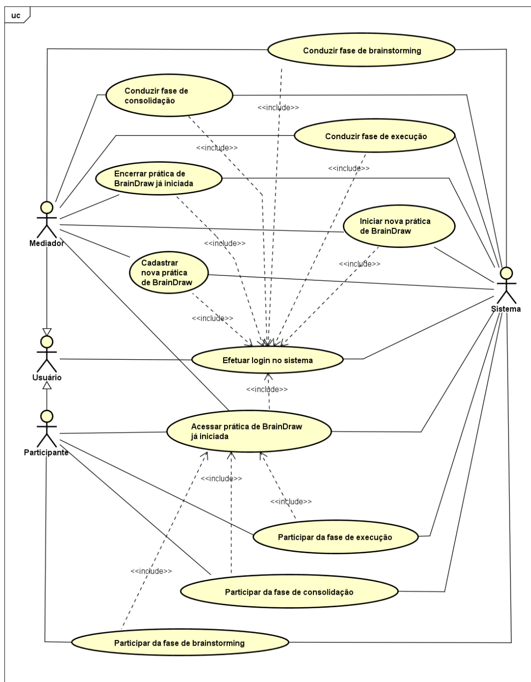
Figura 29 – Diagrama de caso de uso do Sistema DEA
