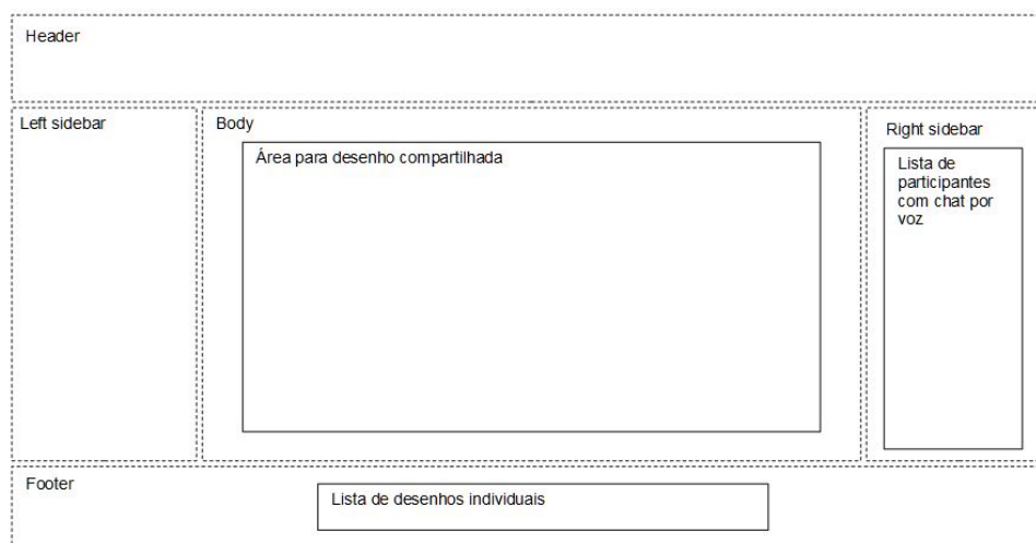
Figura 23 – Oficina C: wireframe referente à IU da fase de consolidação gerado a partir dos desenhos consolidados.
