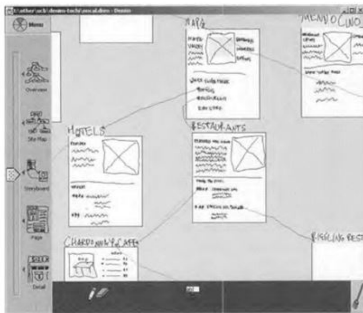
Figura 6 – DENIM – interface de usuário (IU) de visualização do storyboard .
