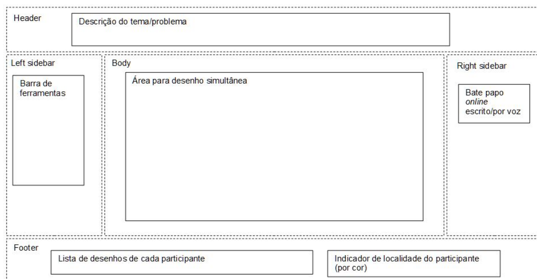
Figura 20 – Oficina B: wireframe referente à IU da fase de consolidação.
