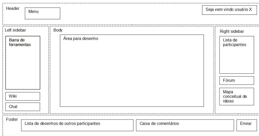
Figura 21 – Oficina C: wireframe referente à IU da fase de execução gerado com os resultados dos desenhos preliminares.
