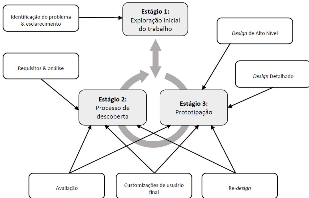
Figura 13 – Mapeamento das fases do ciclo de desenvolvimento de software por estágios da metodologia de DP.
