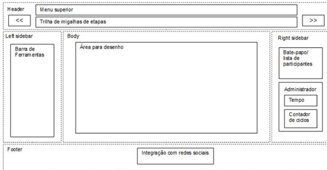
Figura 18 – Oficina A: wireframe consolidado da aplicação.
