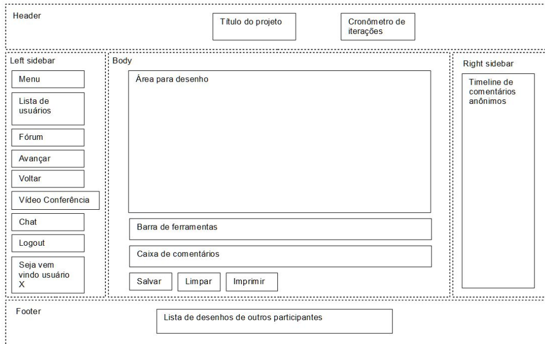
Figura 22 – Oficina C: wireframe referente à IU da fase de execução gerado com os resultados dos desenhos consolidados de todos os grupos.
