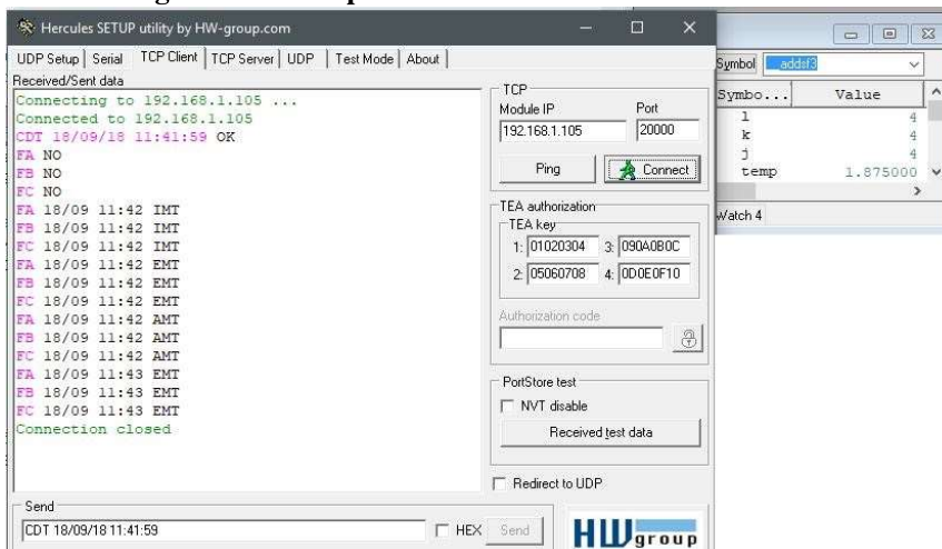
Figura 54: Múltiplos eventos todas as fases - 10 eventos
