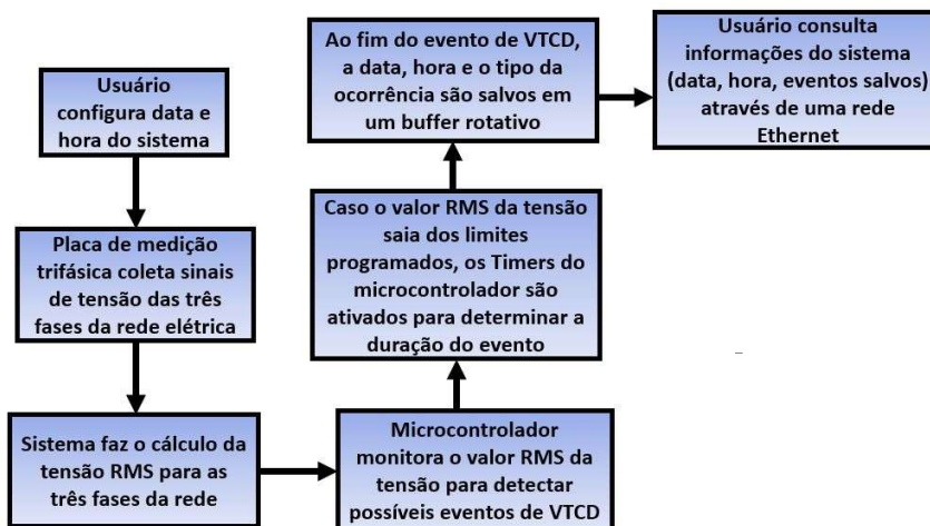
Figura 19: Fluxograma apresentando a sequência de atividades feitas pelo sistema
