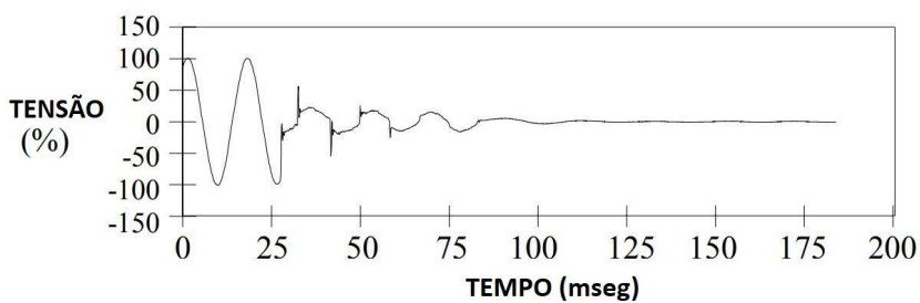
Figura 4: Variação da tensão instantânea durante evento de interrupção
