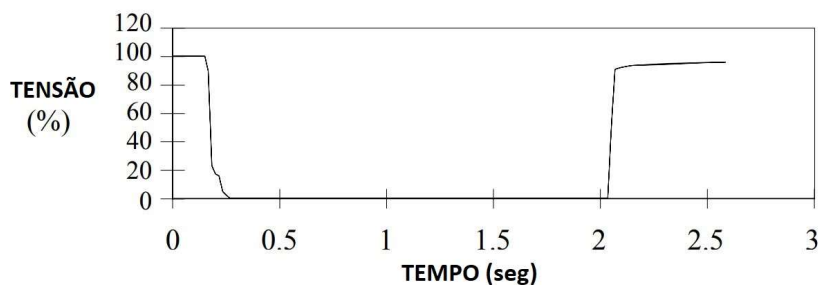
Figura 3: Variação da tensão eficaz durante evento de interrupção
