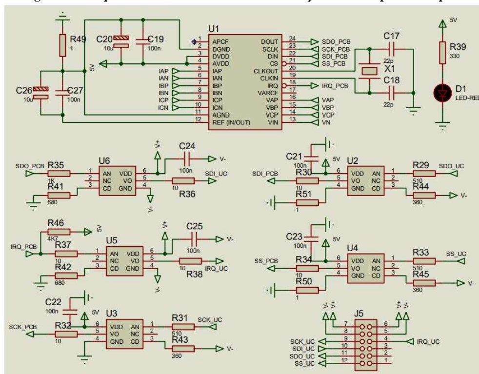
Figura 17: Esquemático da interface de comunicação e dos acopladores ópticos
