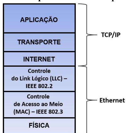
Figura 26: Rede com protocolo TCP/IP e padrão Ethernet
