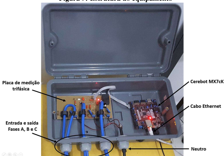
Figura 9: Estrutura do equipamento
