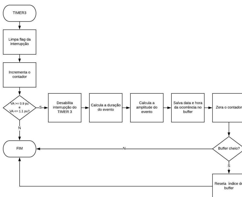
Figura 23: Fluxograma da rotina de tratamento da interrupção do TIMER3
