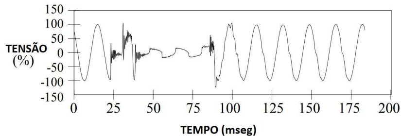
Figura 6: Variação da tensão instantânea durante evento de afundamento
