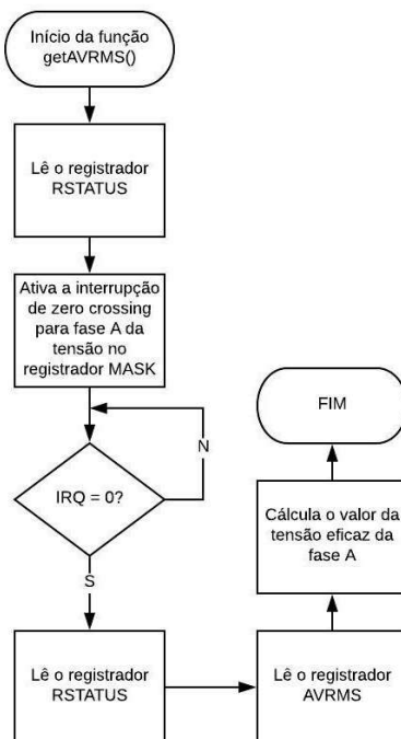
Figura 21: Fluxograma do firmware da função getAVRMS
