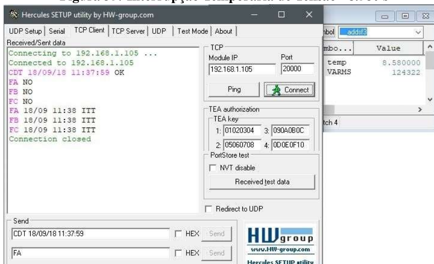
Figura 35: Interrupção Temporária de Tensão - 8.580 s
