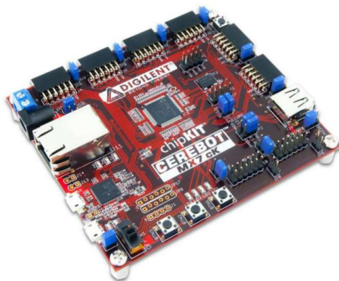
Figura 10: Placa de desenvolvimento Cerebot MX7cK
