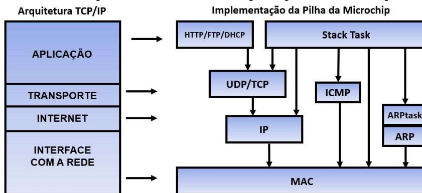
Figura 25: Estrutura da pilha TCP/IP da Microchip comparada com a arquitetura TCP/IP
