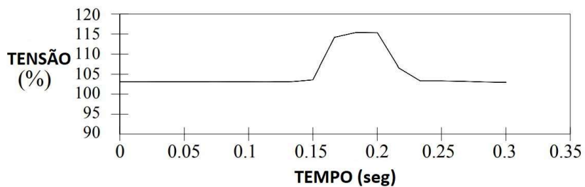
Figura 7: Variação da tensão eficaz durante evento de elevação
