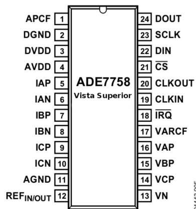
Figura 13: Configuração de pinos do circuito integrado ADE7758
