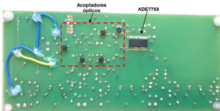
Figura 18: Face inferior da placa de medição trifásica
