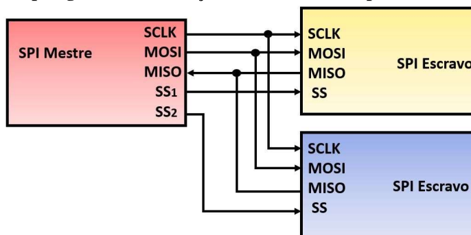
Figura 16: Topologia da comunicação SPI - Um mestre para um ou mais escravos
