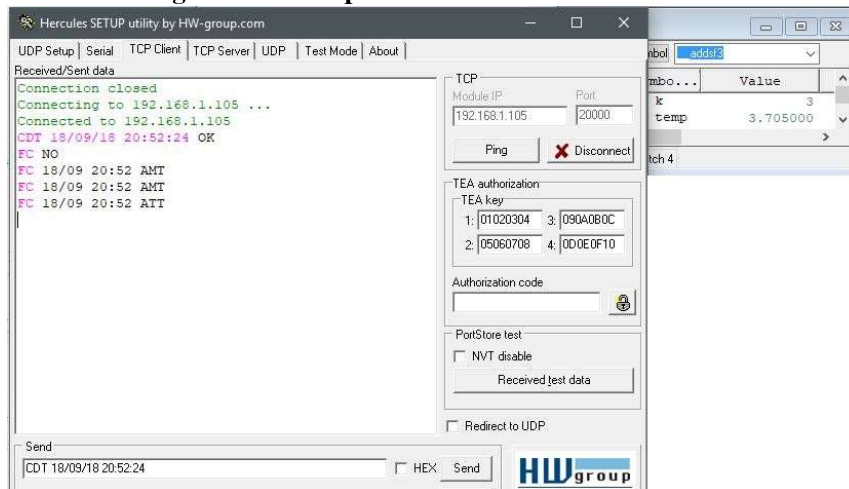
Figura 52: Múltiplos eventos na fase C - 3 eventos
