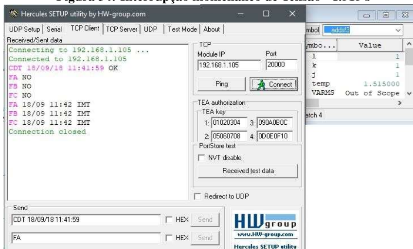
Figura 34: Interrupção momentânea de Tensão - 1.515 s
