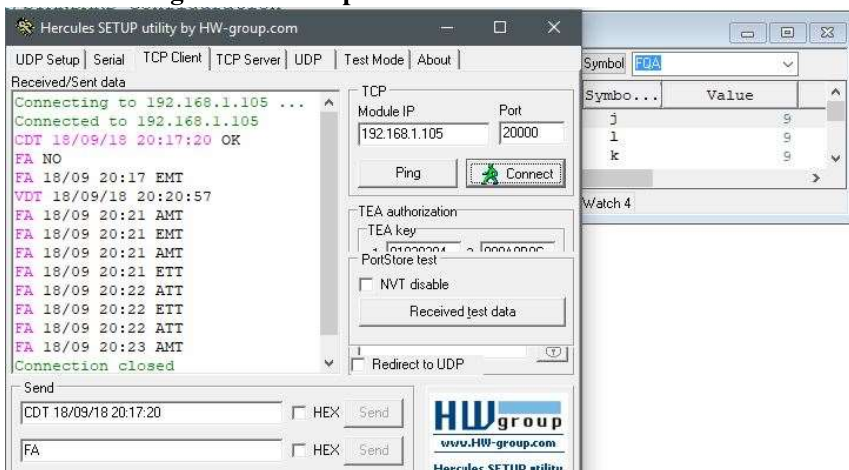
Figura 48: Múltiplos eventos na fase A - 9 eventos
