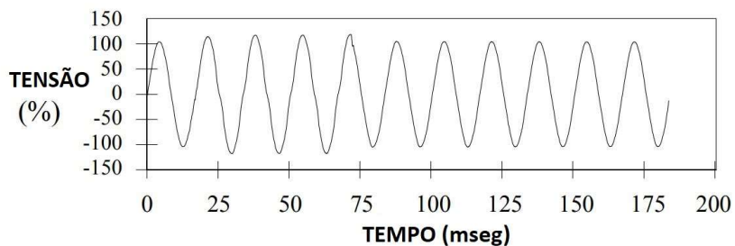
Figura 8: Variação da tensão instantânea durante evento de elevação
