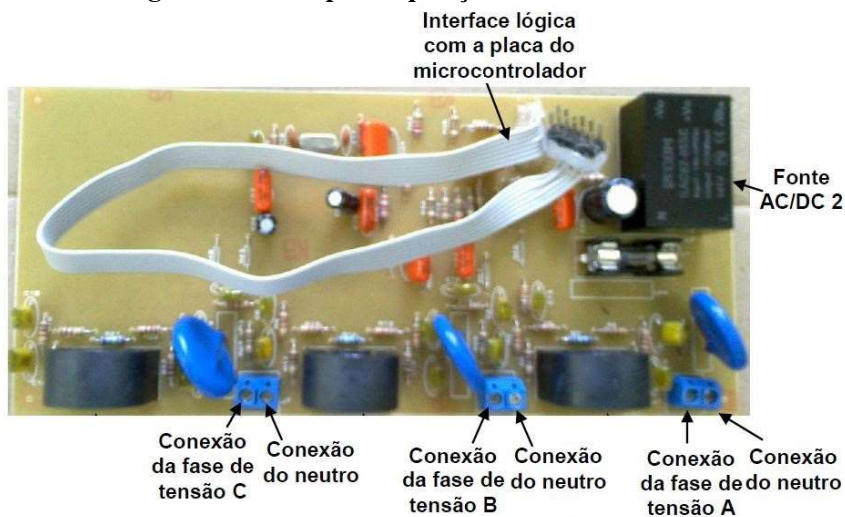
Figura 12: Placa para aquisição dos sinais de tensão
