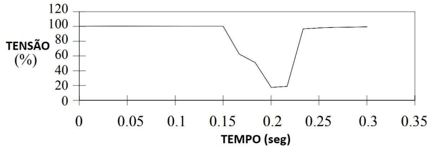
Figura 5: Variação da tensão instantânea durante evento de afundamento
