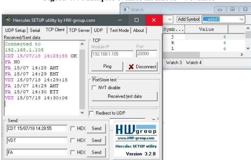
Figura 47: Múltiplos eventos na fase A - 4 eventos
