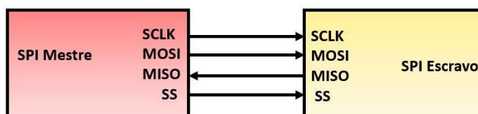
Figura 15: Topologia da comunicação SPI - Um mestre e um escravo
