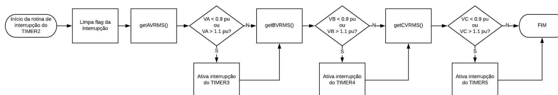
Figura 22: Fluxograma da rotina de tratamento da interrupção do TIMER2
