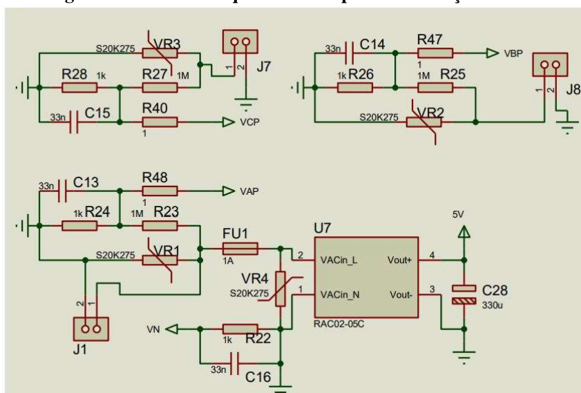
Figura 14: Parte do esquemático da placa de medição trifásica
