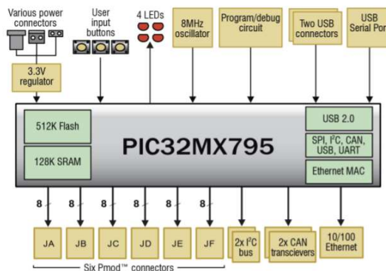
Figura 11: Diagrama do circuito da placa Cerebot MX7cK
