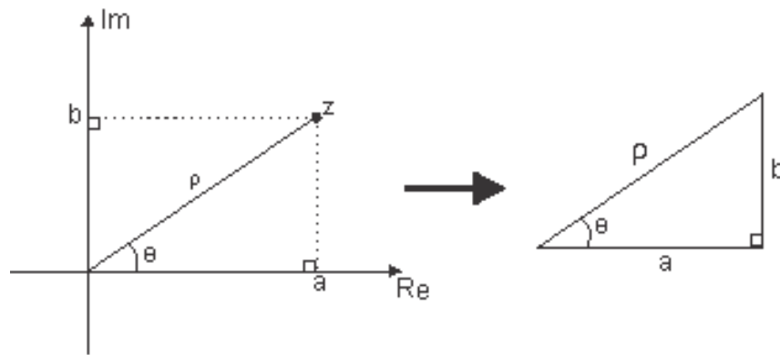
Figura 3: Representação Geométrica
