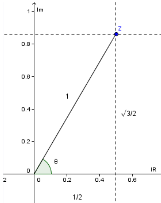
Figura 79: Representação geométrica
