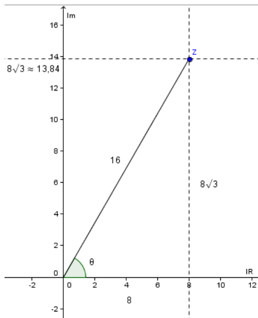
Figura 72: Representação geométrica
