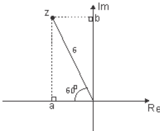
Figura 45: Representação geométrica
