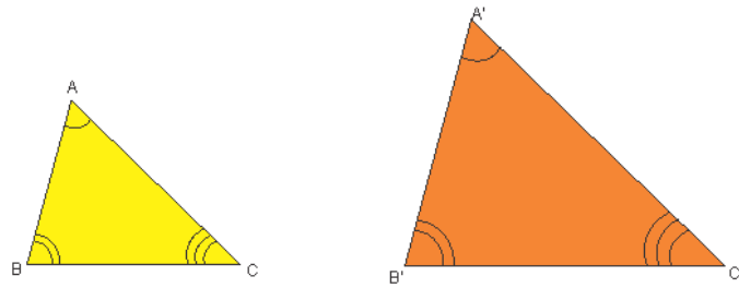
Figura 10: Triângulos semelhantes
