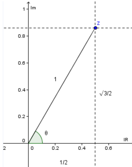
Figura 78: Representação geométrica
