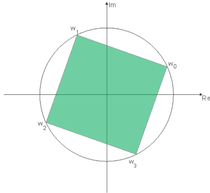
Figura 6: Raízes Quartas
