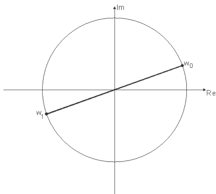
Figura 4: Raízes Quadradas
