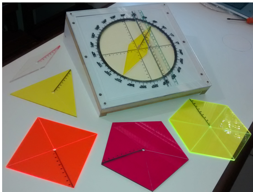
Figura 38: GeoPlexo completo
