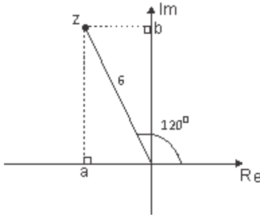
Figura 44: Representação geométrica
