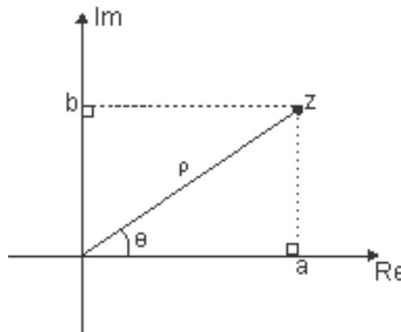
Figura 7: Representação Geométrica
