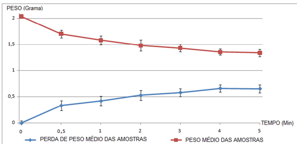
Figura 6 – Comportamento de queda média de peso das amostras sob compressão e peso médio do líquido exsudado
