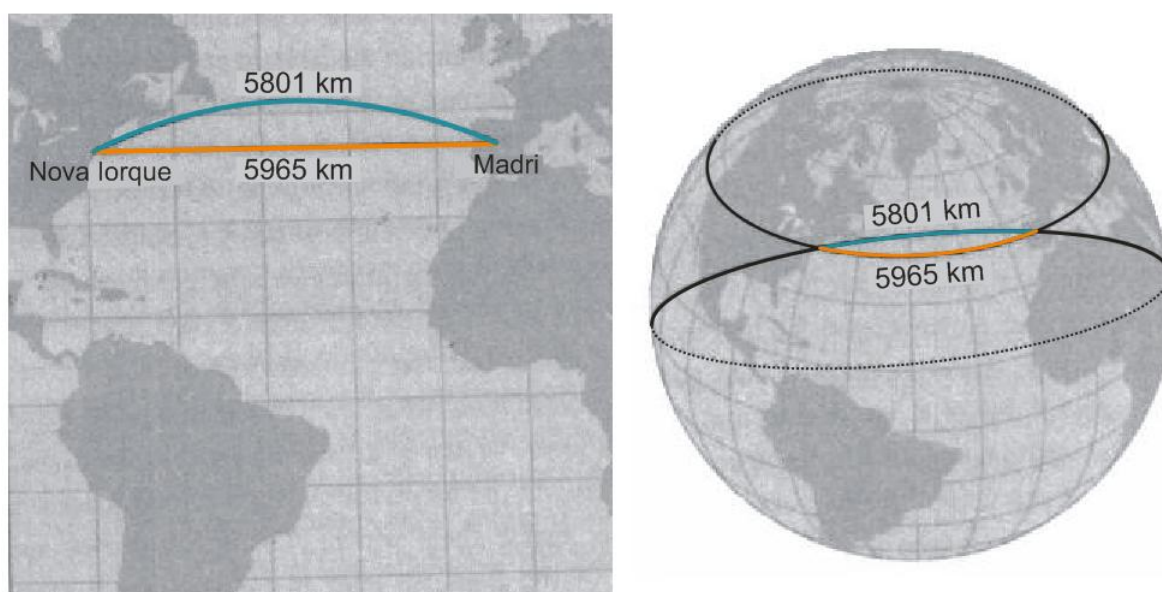
Figura 38: Representação das distâncias entre Nova Iorque e Madri, pelo paralelo e pela geodésica.
