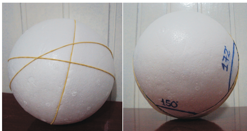
Figura 27: Representação dos triângulos com somas próximas dos valores mínimo e máximo.
