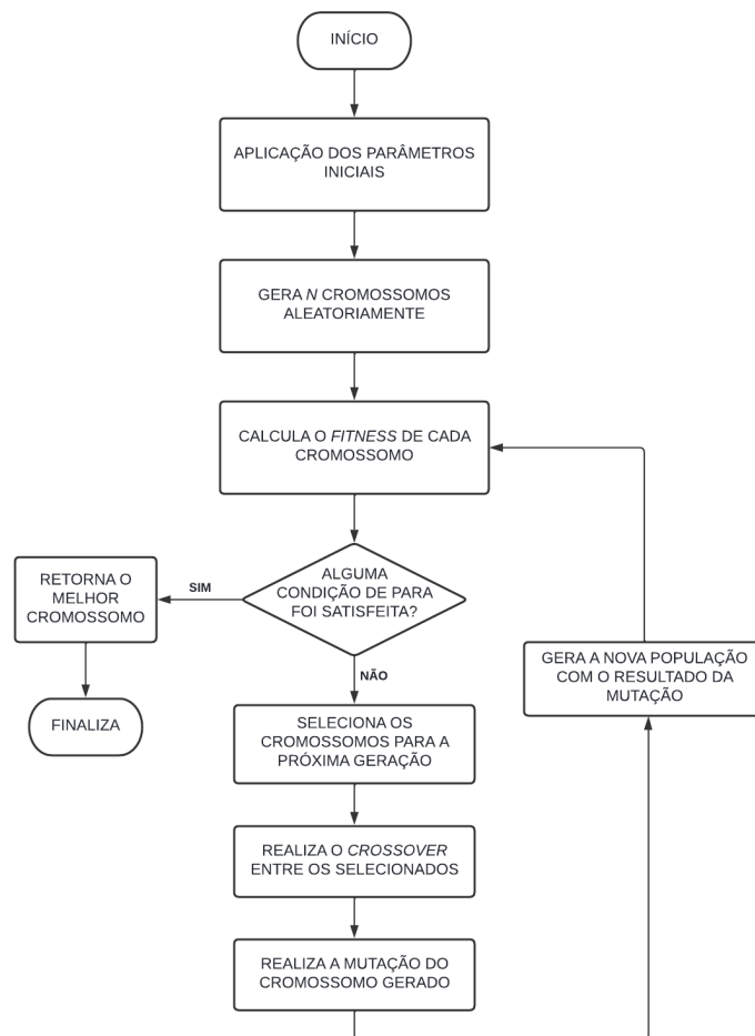
Figura 2 – Diagrama de execução do AG
