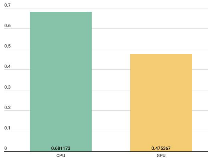
Figura 8 – Tempos para execução apenas da distância Euclidiana do dataset ATT48 (ms)
