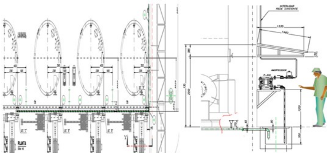
Figura 9 – Detalhamento do projeto- Planta do circuito fechado Fonte: Empresa
